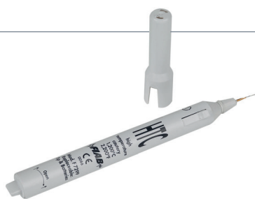
Cauterizador REUTILIZABLE Mod F2799. Alta temperatura (1200°) Con pilas (2xAA) y punta desechable. 7389000
