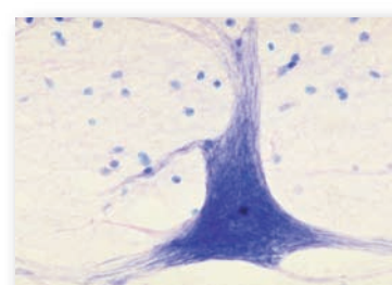
Microfotografía de neurona. Las dendritas de las neuronas son las conexiones de entrada, mientras que los axones son las salidas, por donde se envían impulsos o señales a otras células.
