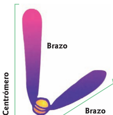
Estructura de un cromosoma
